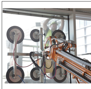
Smartlift SL808 bei der Fenstermontage
